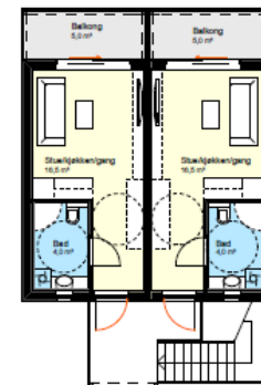
2.ETASJE
