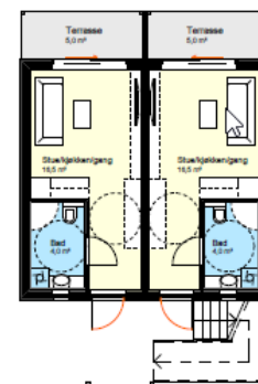
1.ETASJE
