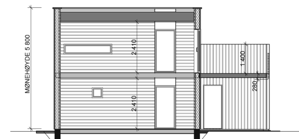
SNITT
