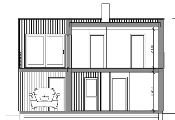
Snitt
